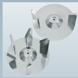
Стандартная крыльчатка, нержавеющая сталь 6-ти лопастная 548 000 9305 Двойная крыльчатка, нержавеющая сталь 2-х лопастная 548 000 3501 Крыльчатка для перетирания, нержавеющая сталь, 2-х лопастная 548 000 3400
