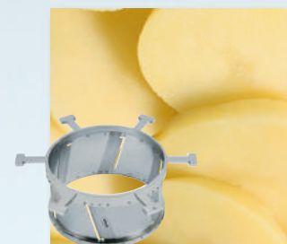
Цилиндр для нарезки, нержавеющая сталь 1,5 мм, зубчатый с 6 ножами 548 100 3815 2 мм, зубчатый с 6 ножами 548 100 3820 2,5 мм, зубчатый с 6 ножами 548 100 3825 4 мм, гладкий с 6 ножами 548 100 3840 6 мм, гладкий с 6 ножами 548 100 3860
