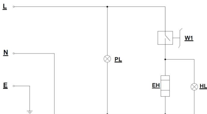
Рис 3 Электросхема для модели DF-81
