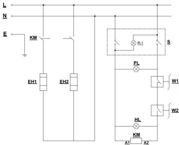
Рис 4 Электросхема для модели DF-20L
