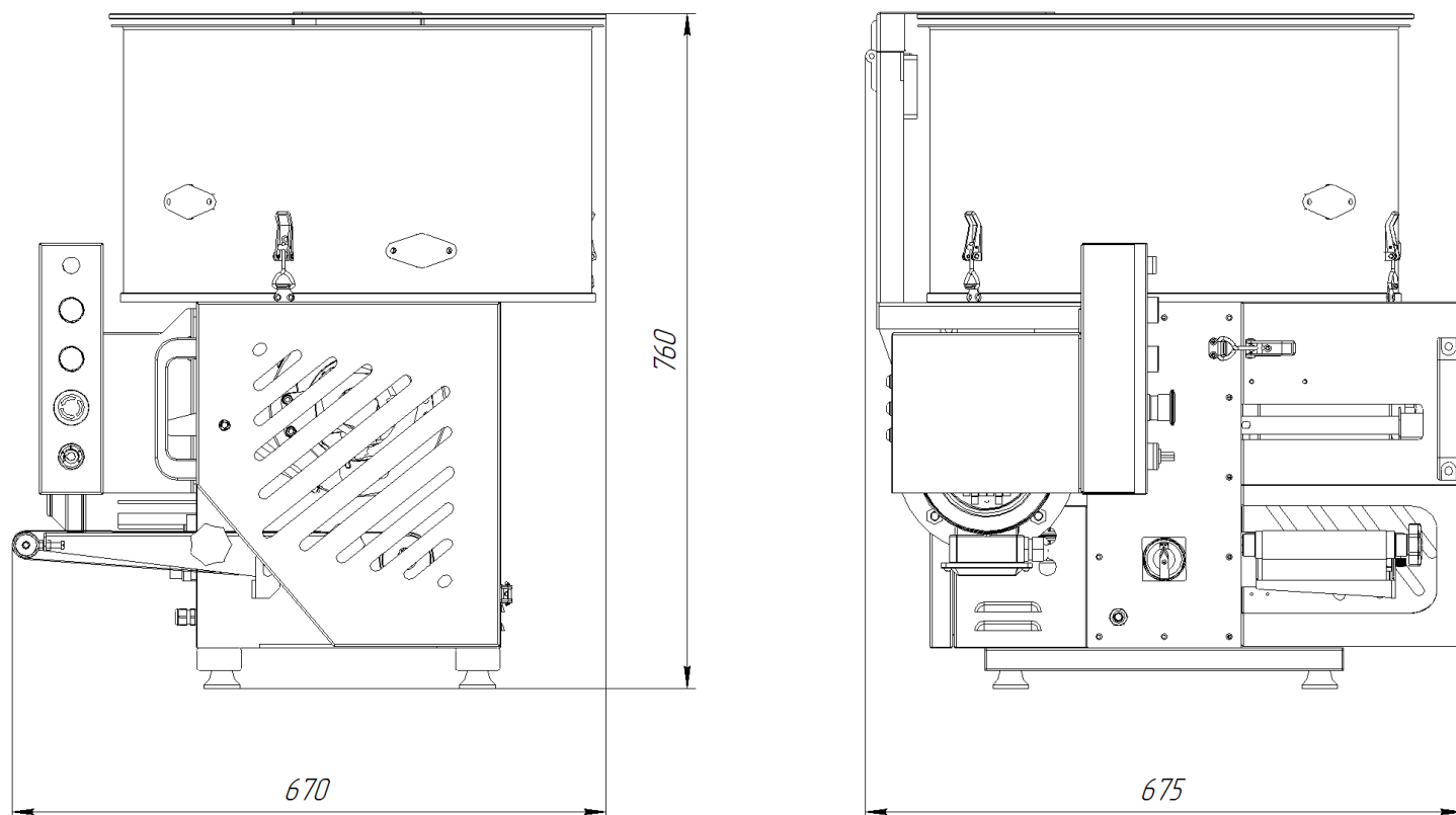
Рис.1 Габаритные размеры
