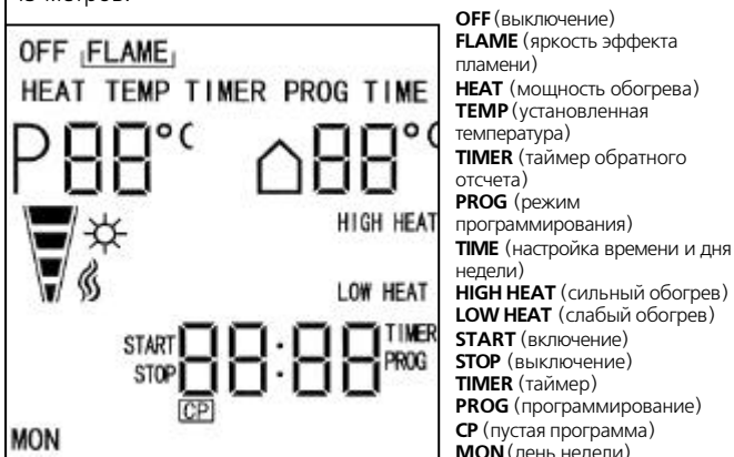
Иллюстрация 8 - жидкокристаллический дисплей
