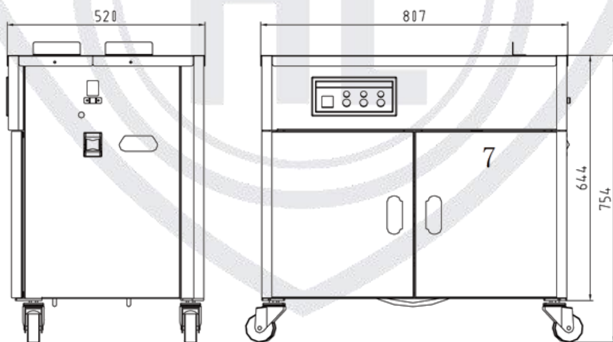
Рис. 4 Габаритные размеры AS-10N
