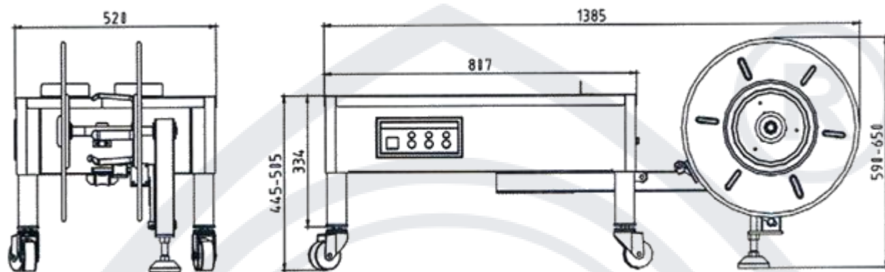
Рис. 6 Габаритные размеры AS-13N
