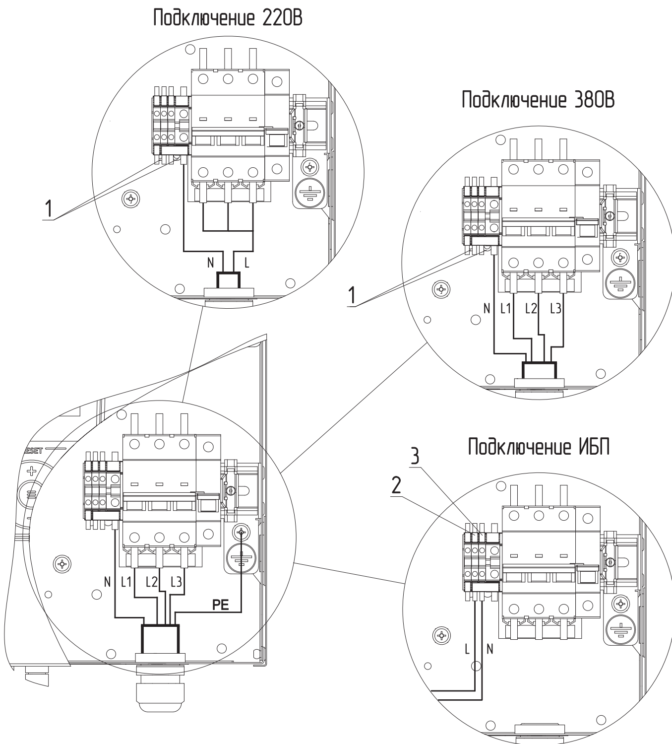
Рис.4 Схема подключения электрического котла ZOTA LUX-X 4,5-48 кВт
