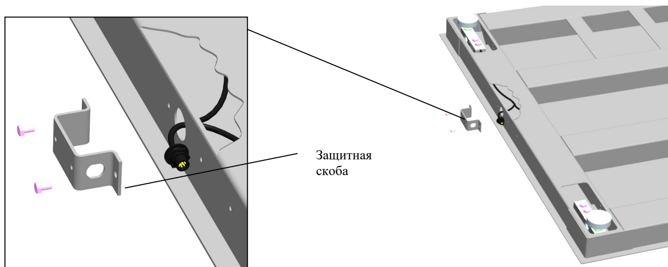
Рис. 2а. Подготовка модуля
