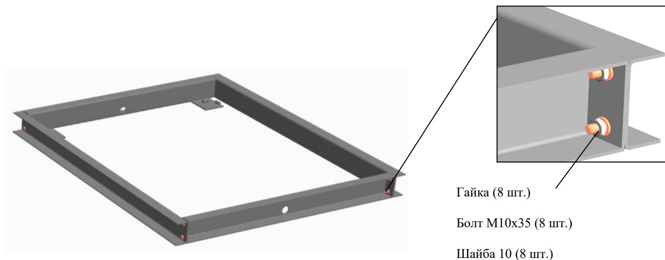
Рис.3. Сборка рамы
