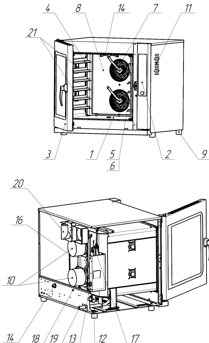
Рис.3 Общий вид пароконвектомата PR-SIW-06.
