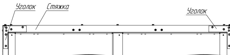
Рис.2 Установка стяжки (Вид изнутри шкафа)
