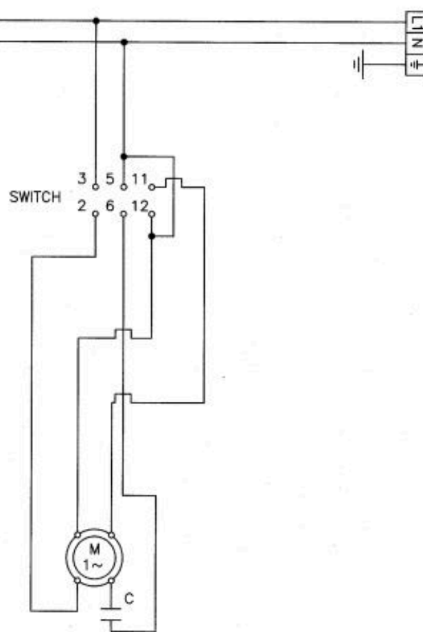
Однофазное соединение AB.22/AT - TR.22/TS - TR.32/TS
