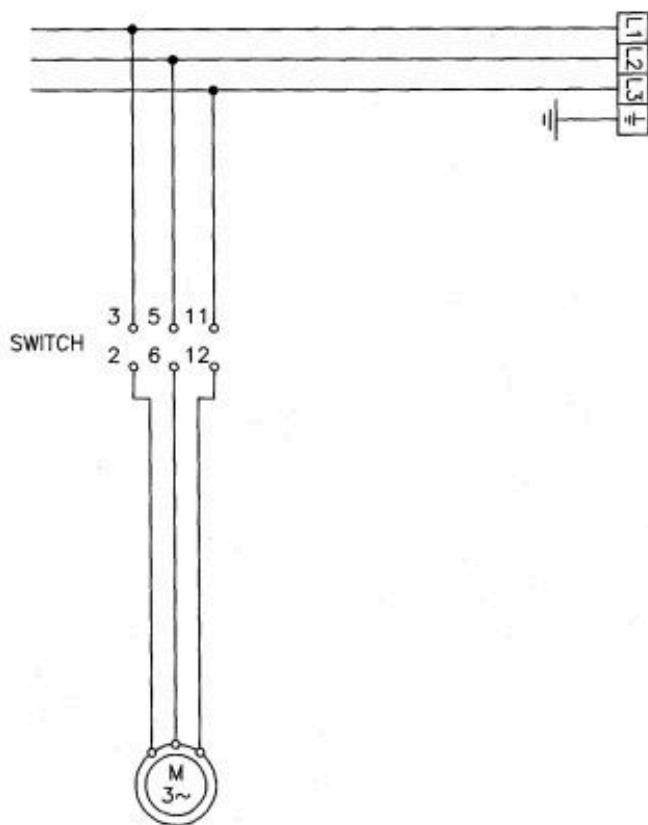
Трехфазное соединение AB.22/AT - TR.22/TS - TR.32/TS
