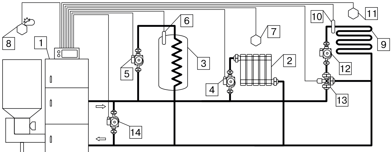
Рис.25 Схема подключения с узлом рециркуляции для котлов с контроллером ZOTA серии I-Line 223 SFA (для ZOTA Twist, Stahanov, Pellet S, Maxima, Robot, Стаханов, Pellet A, Optima, Pellet Pro)
