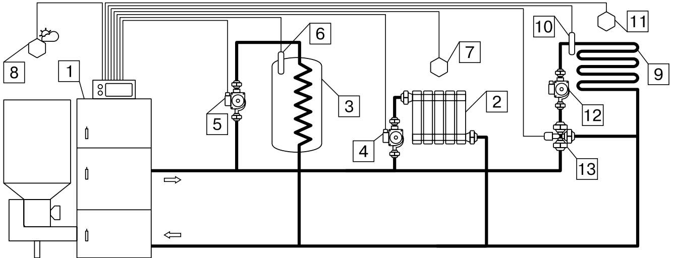
Рис.24 Схема подключения котлов с контроллерами ZOTA серии R-Line 230 SFA (для ZOTA Twist Plus, Stahanov Black 16-65кВт, Pellet Black) и ZOTA I-Line 223 SFA (для ZOTA Twist, Stahanov, Pellet S, Maxima, Robot, Стаханов, Pellet A, Optima, Pellet Pro)
