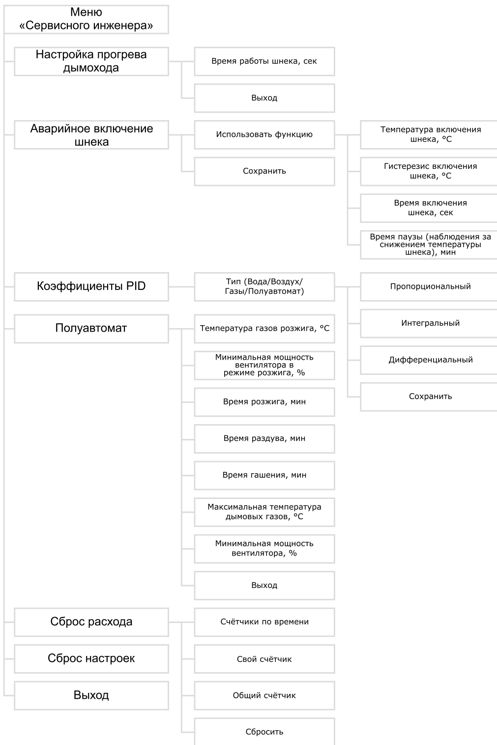
Рис.23 Блок-схема меню сервисного инженера (продолжение)
