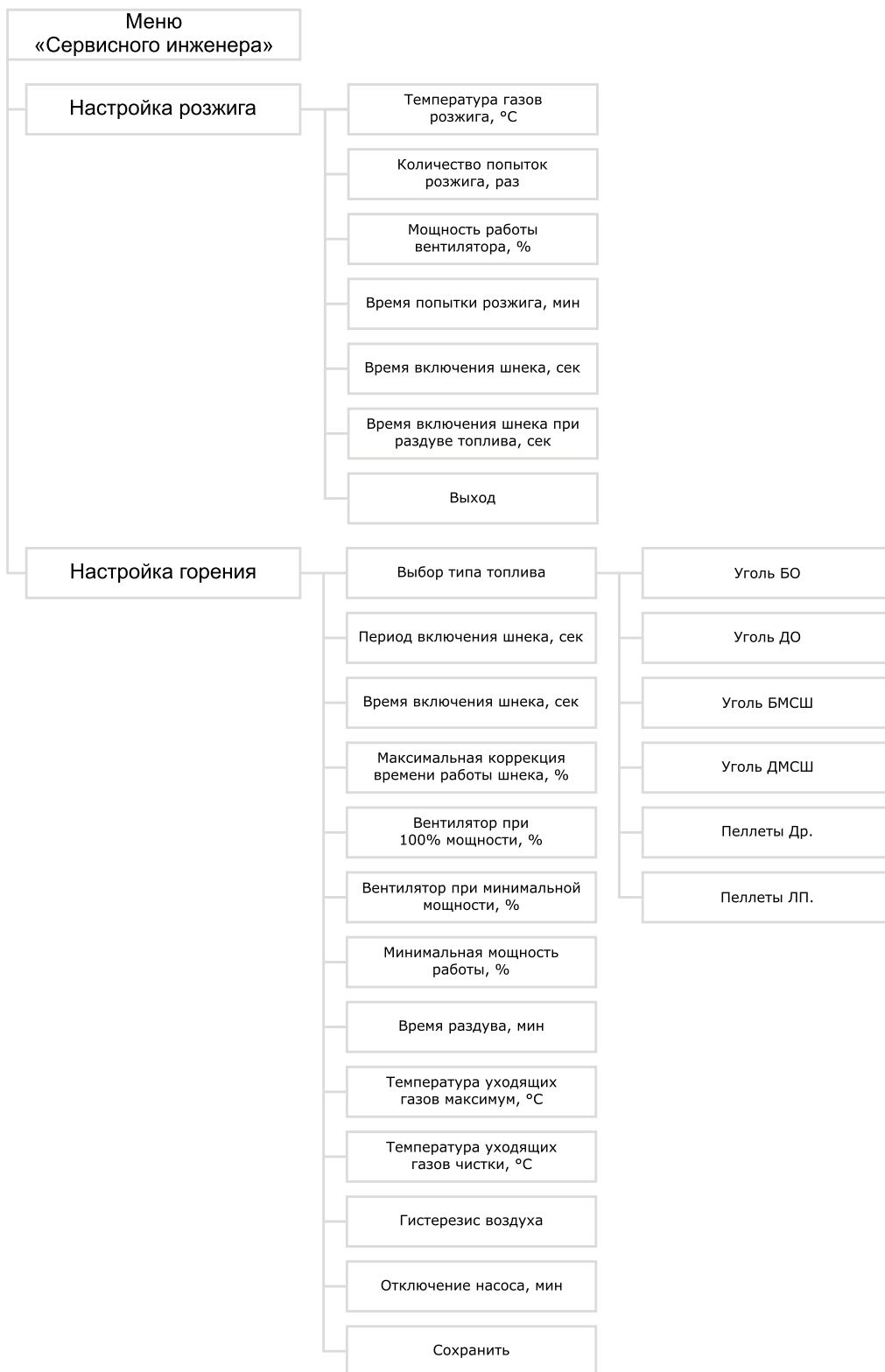
Рис.22 Блок-схема меню сервисного инженера (продолжение)
