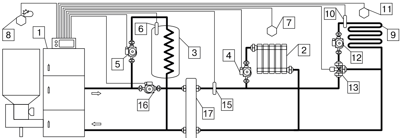
Рис.26 Схема подключения с гидроразделителем, контуром ГВС и теплого пола для котлов с контроллером ZOTA серии I-Line 223 SFA (для ZOTA Twist, Stahanov, Pellet S, Maxima, Robot, Стаханов, Pellet A, Optima, Pellet Pro)
