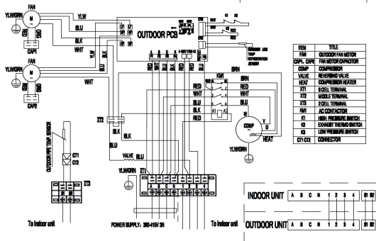
Схема для наружных блоков (Модель LAC-60T)
