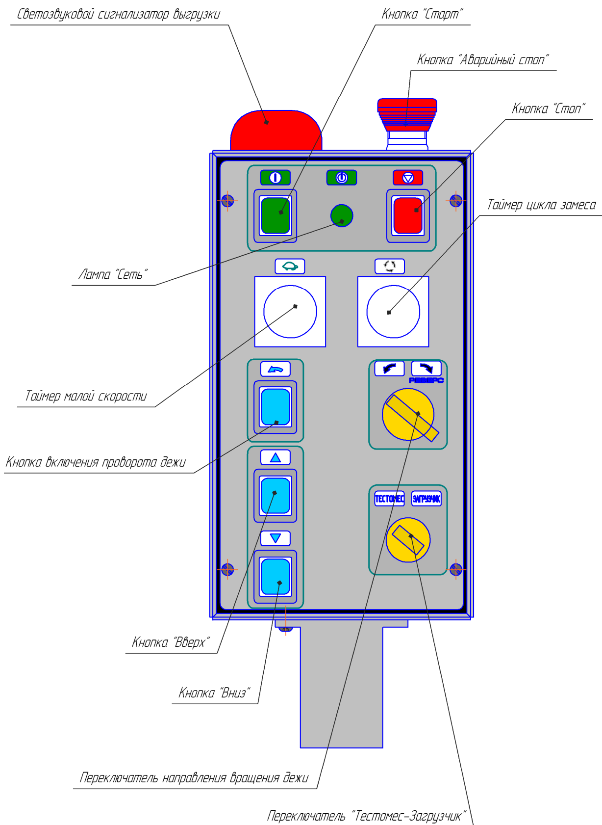
Рисунок 2 – Пульт управления машины.
