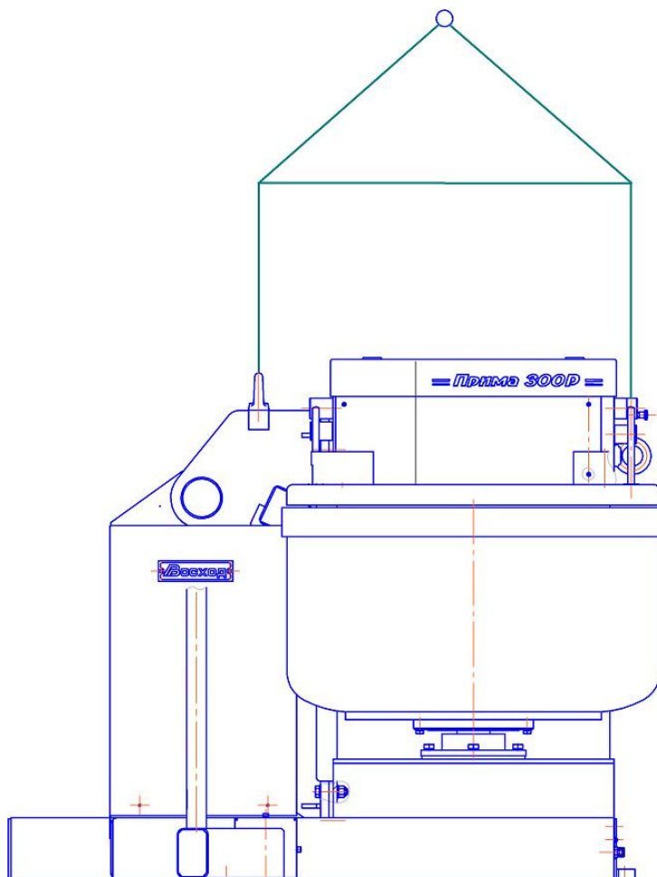
Рисунок 7 – Схема строповки машины.
