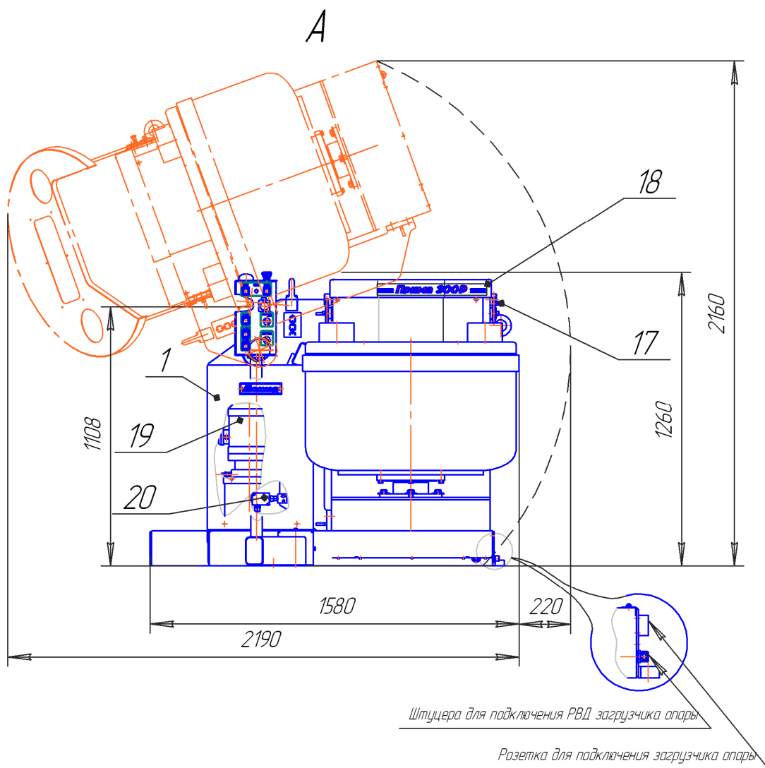
Рисунок 1 – Общий вид машины
