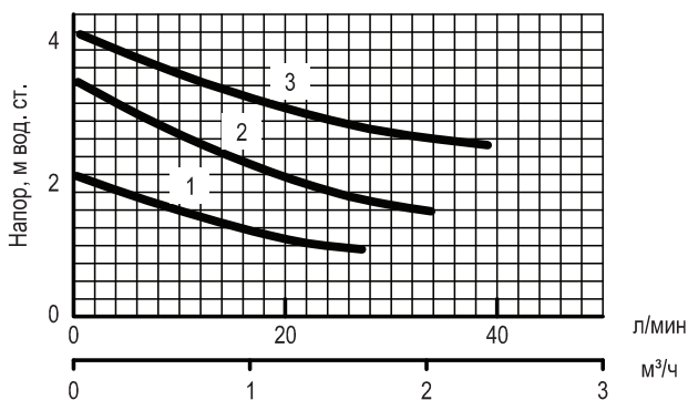
Диаграммы характеристик насосов АСР 25-40, АСР 32-40
