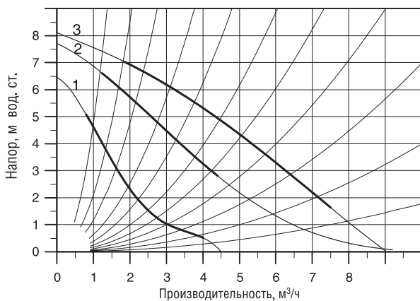
Диаграммы характеристик насоса АСР 25-80
