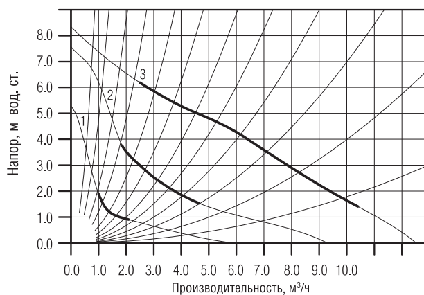
Диаграммы характеристик насоса АСР 32-80
