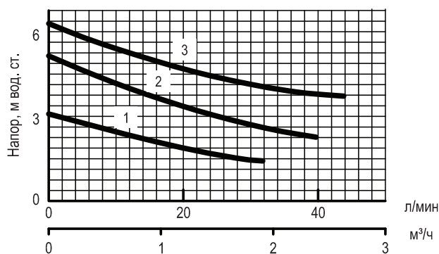
Диаграммы характеристик насосов АСР 25-60, АСР 32-60
