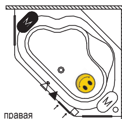
Расположение массажной системы
