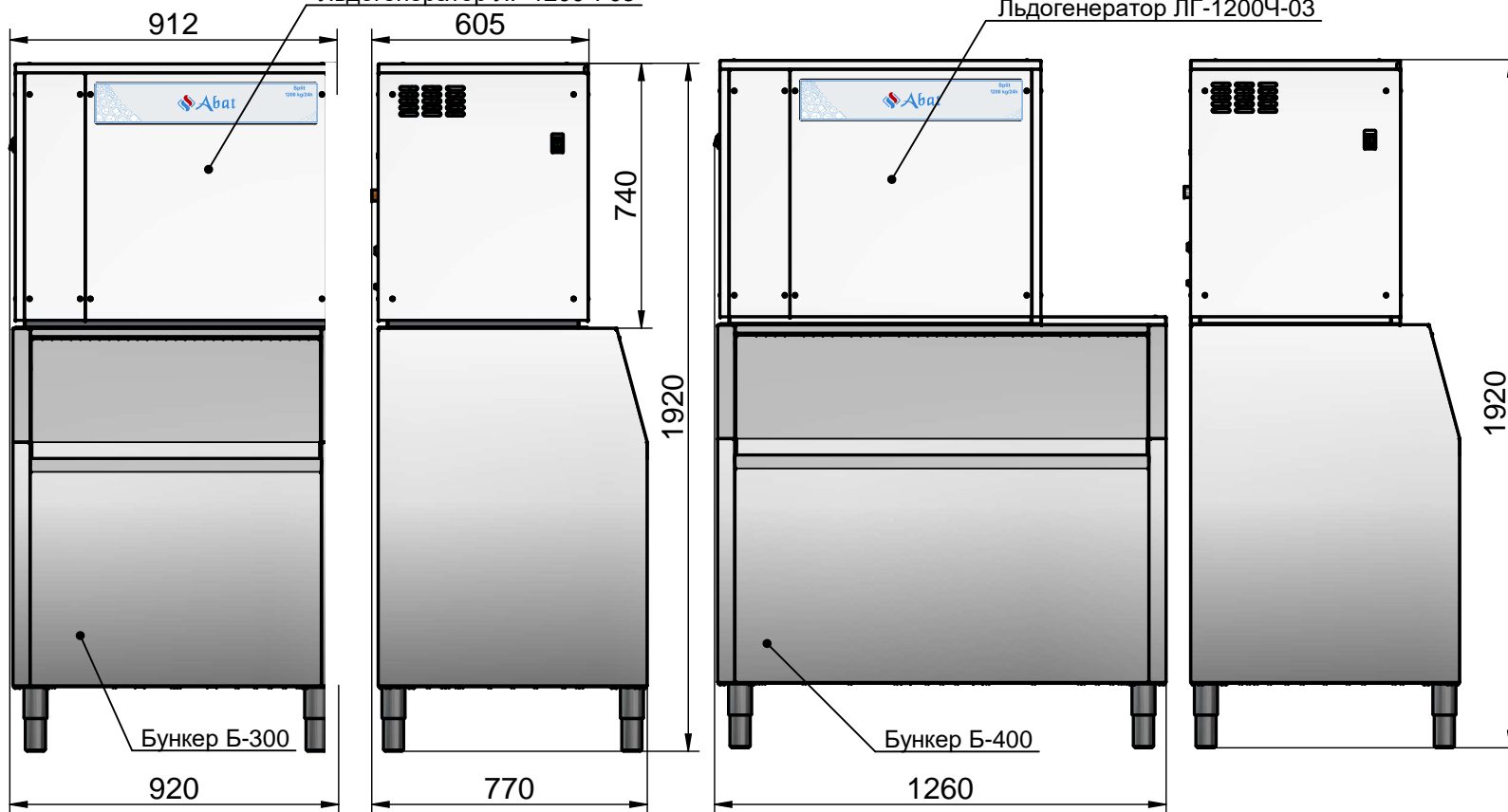
Льдогенератор ЛГ-1200Ч-03
