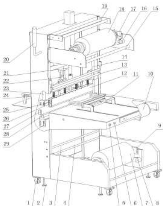
Рис. 1 – Общий вид
