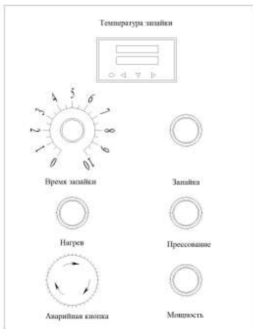
Рис. 2 – Панель управления
